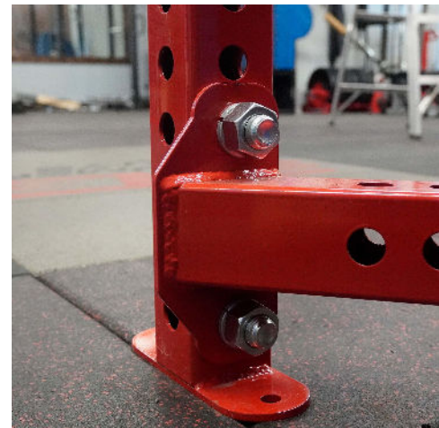
Bolt tabs
